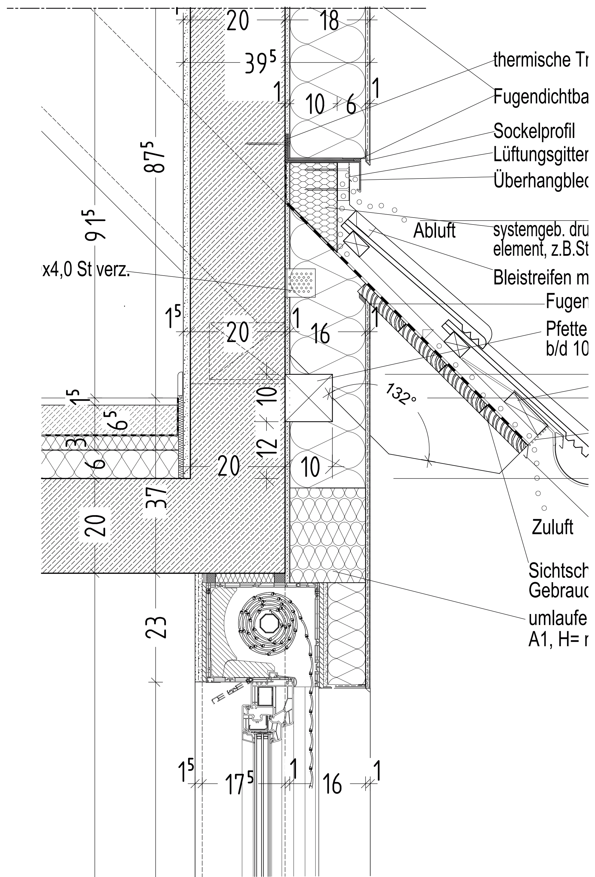
Ausschnitt B 1 M 1 : 5
