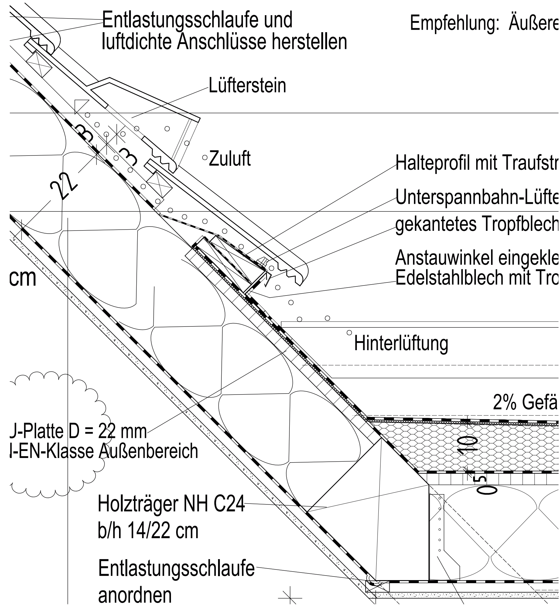
Ausschnitt B 1 M 1 : 5
