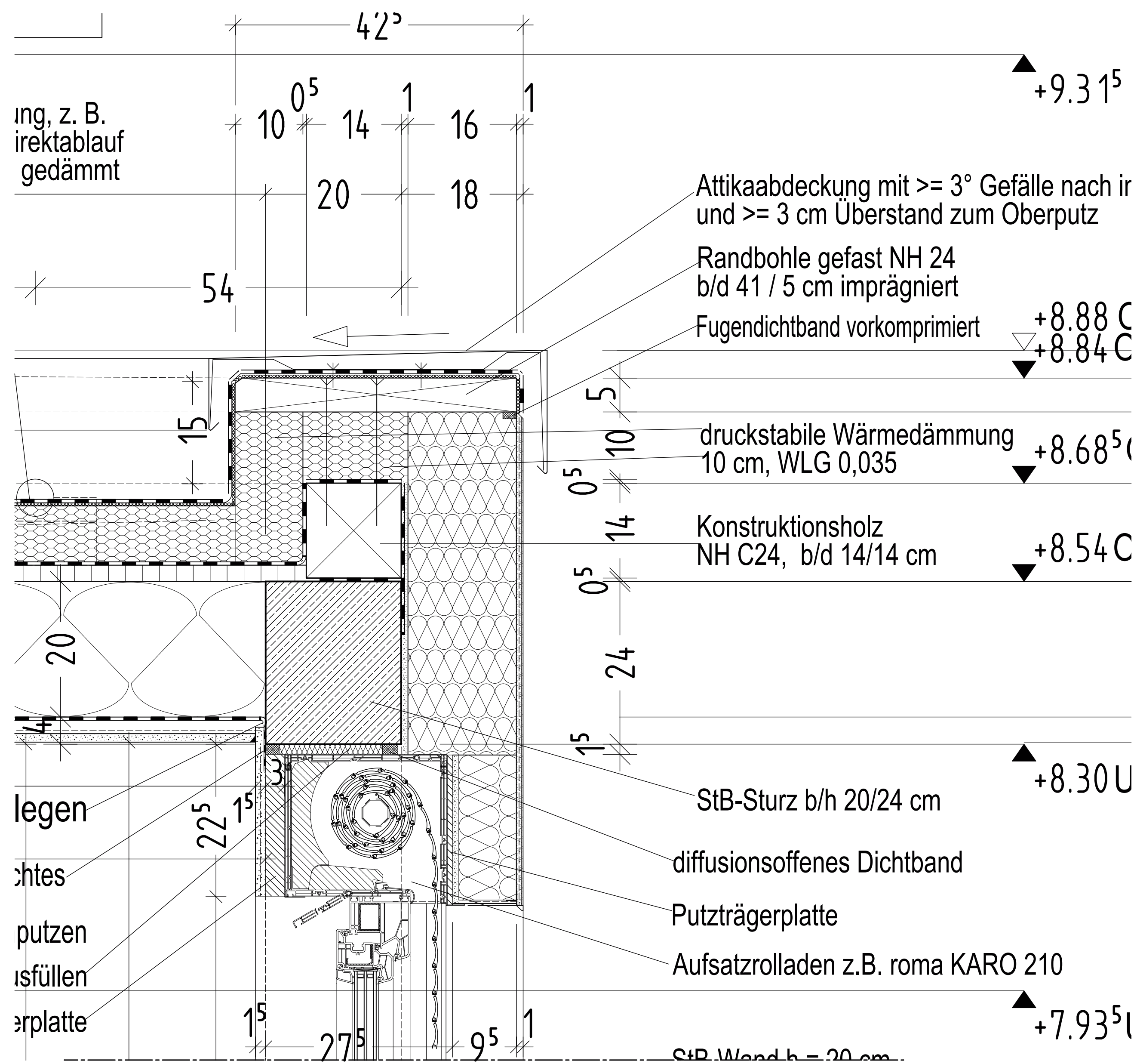
Ausschnitt B 1 M 1 : 5
