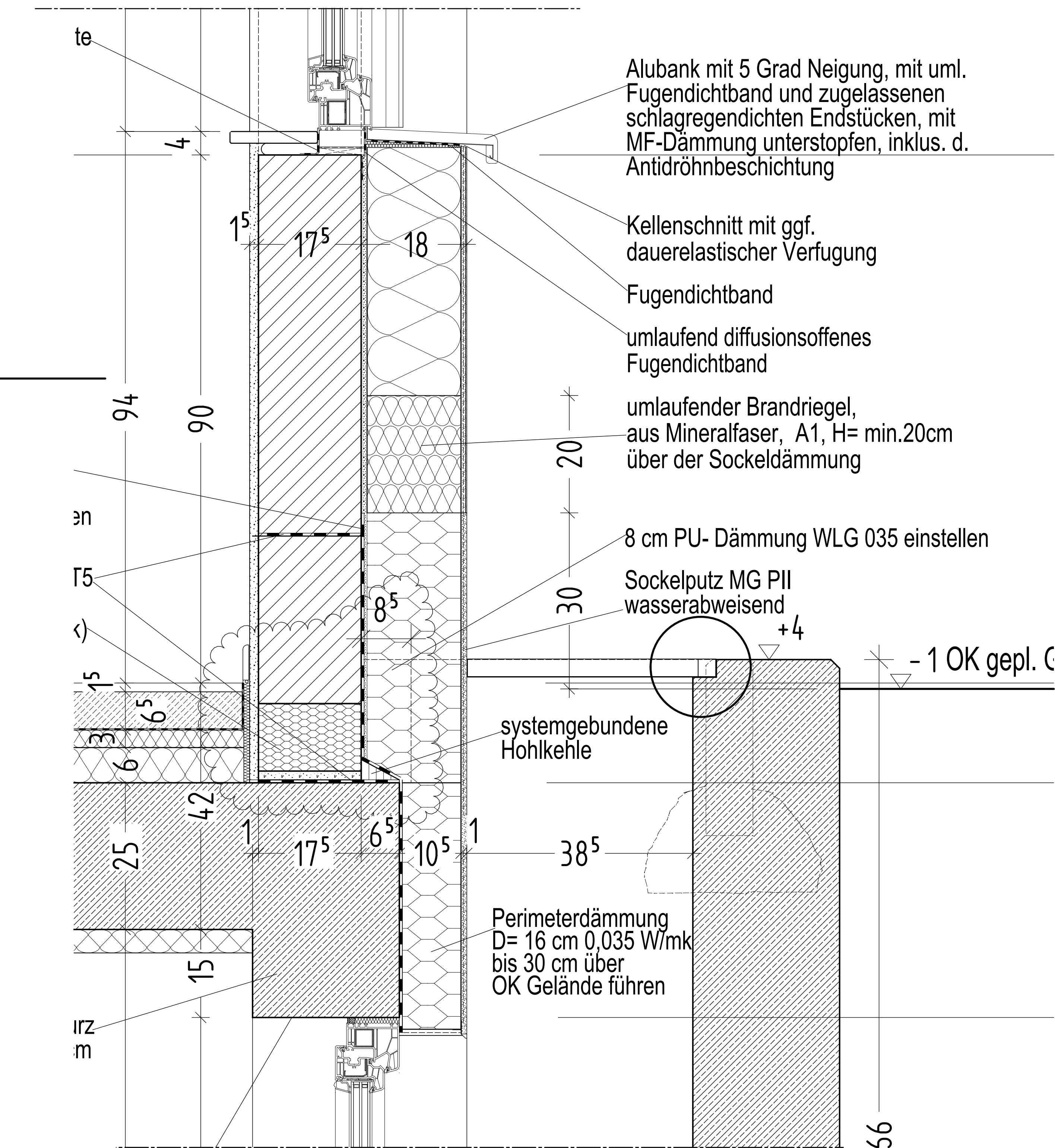
Ausschnitt B 1 M 1 : 5
